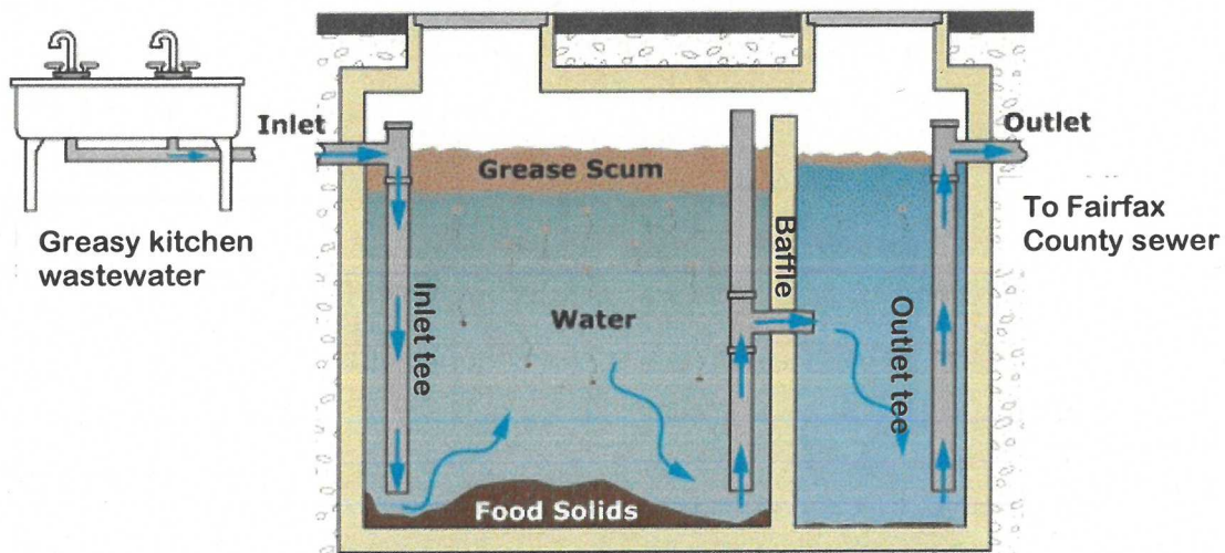
油脂拦截装置示意图
