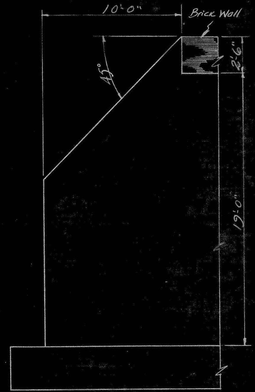
VIEW EE Scale: \frac{1}{4}'' = 1'-0''
