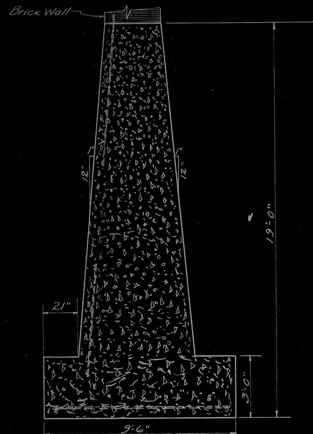
SECTION DD Scale: \frac{3}{8}'' = 1'-0''
